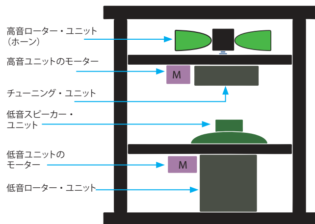
ロータリー・ブロック図
